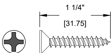
8 - #12 X 1-1/4\"/>
