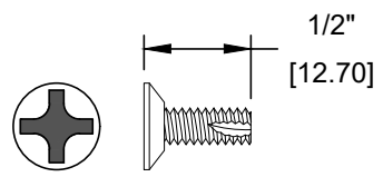
8 - M5 X 1/2" SCREW
